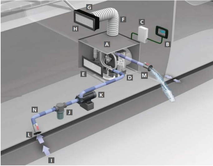
BlueCool S Serisi Paket Klima Montaj Detayı
